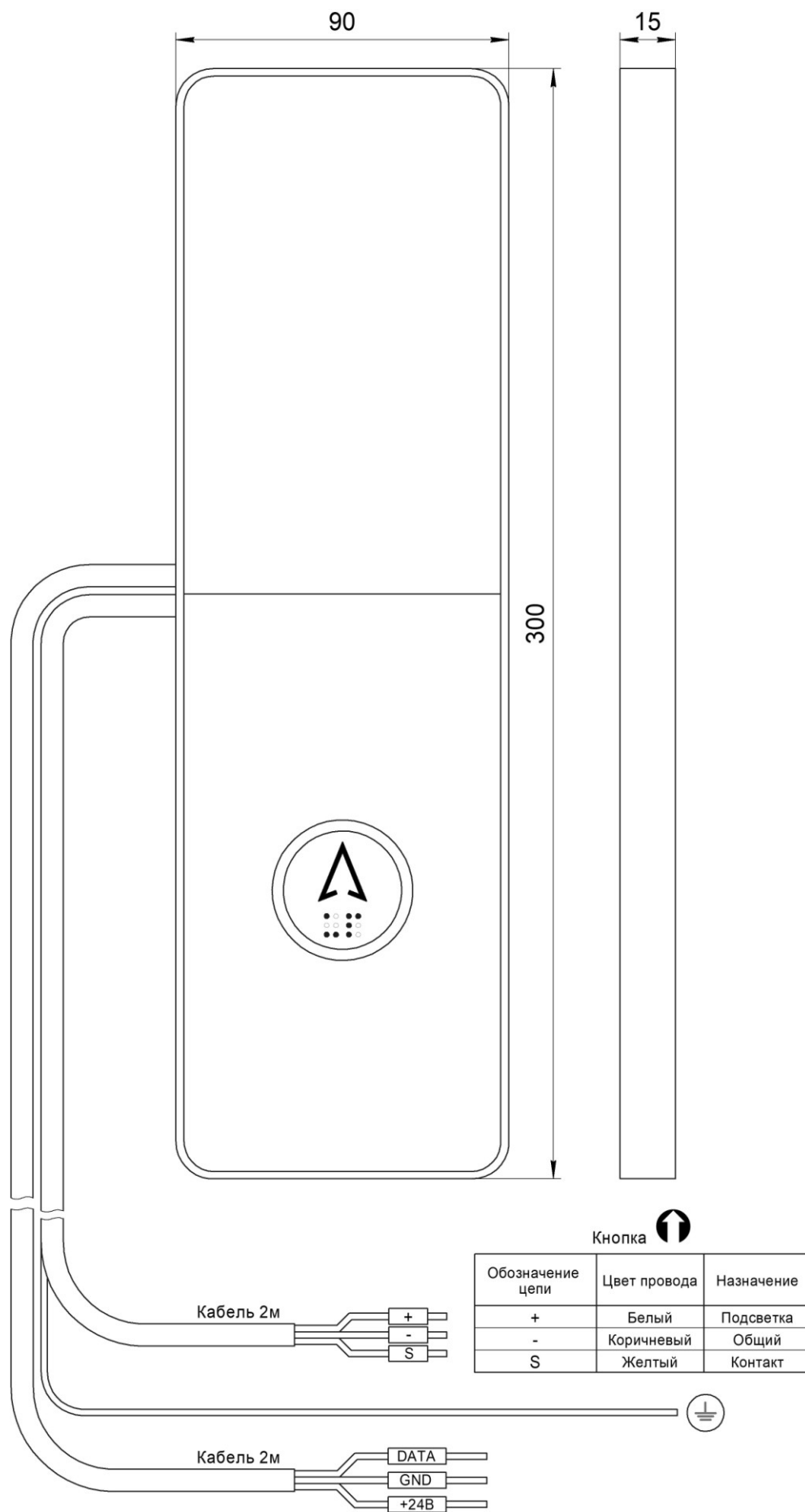
Рис.1 Внешний вид Вызывной пост ОПАЛ НШЕК.468381.030
